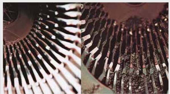
Ein Unterschied wie Tag und Nacht im Kessel: links im Gebrauch mit EcoPlus, rechts mit Standard-Heizöl
